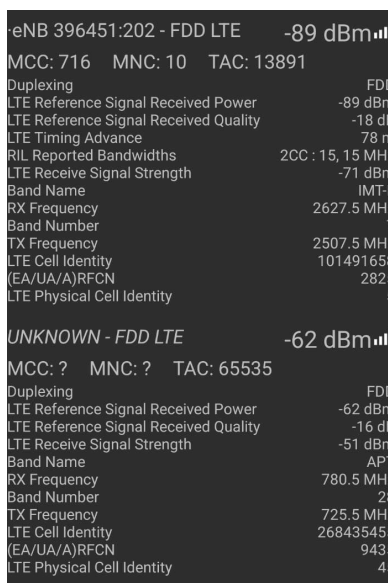
Figura 04. Captura de parámetros LTE obtenidos mediante CellMapper
